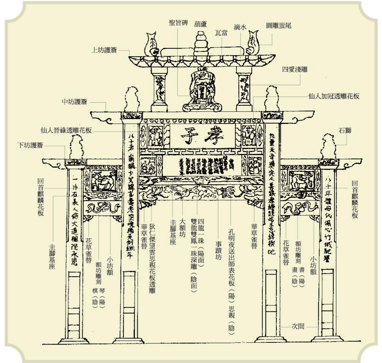
《李錫金孝子坊立面圖》
